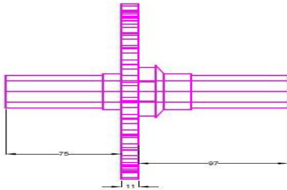
Fig. 1: Sprocket.
